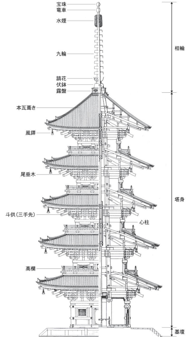
【오층탑 입면도/단면도】
