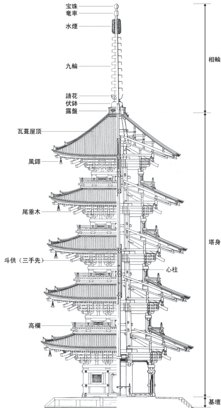
【五重塔 正面图/断面图】
